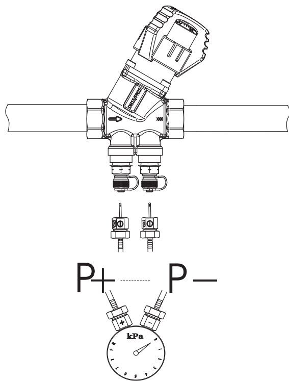
Medición de la presión diferencial de la válvula
